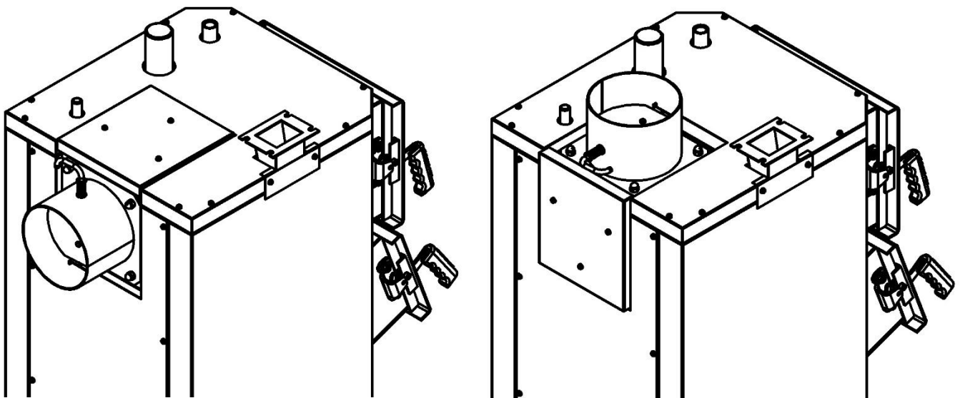
Рисунок 5.2 – Конфігурації встановлення димохода
