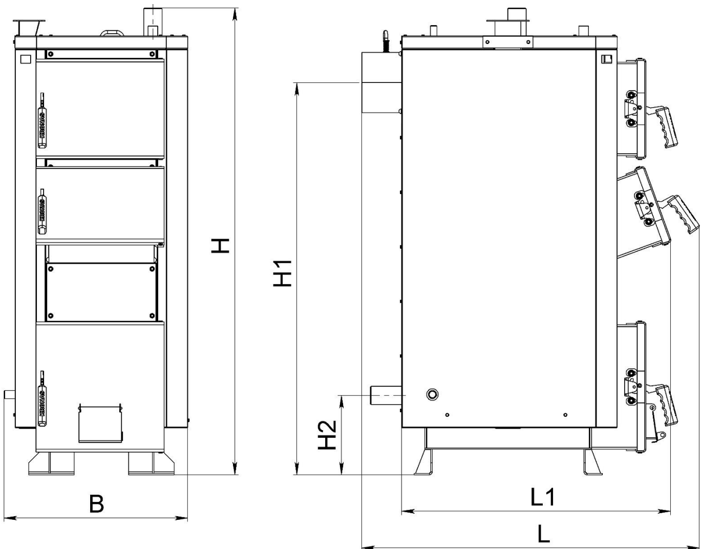
Рисунок 3.1 – Позначення габаритів котла типу КТК
